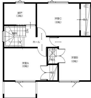
2階 平面図
