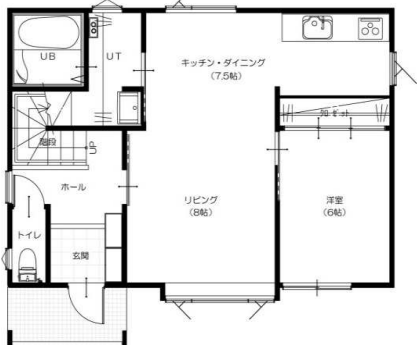
1階 平面図
